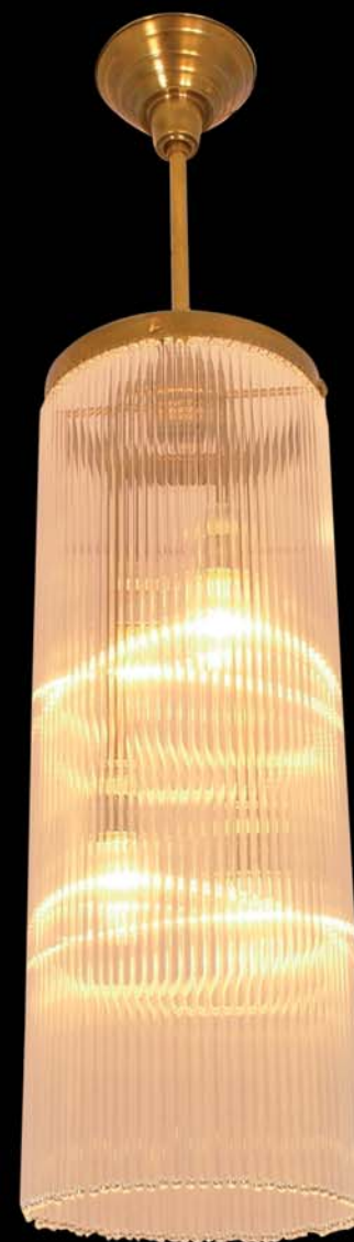
Pendant V. ↑↓ 80 cm ↔ 20 cm 4 x 60 W E14 1 Kg
